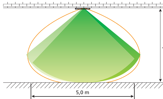
Vista frontale (versioni con MW)
